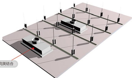
中字铝大梁暗龙骨吊顶系统-三维效果图
