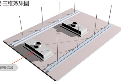
C型暗龙骨吊顶系统-三维效果图
