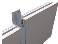
对夹式可拆隔墙搭接
